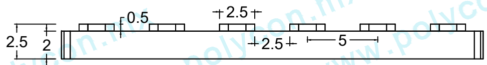
VISTA LATERAL
