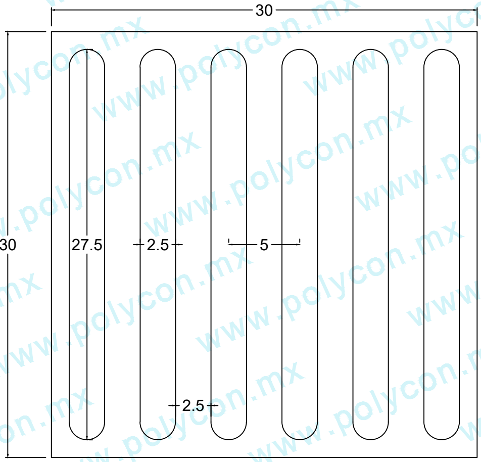
VISTA SUPERIOR
