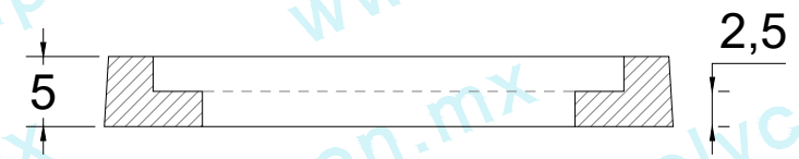
CORTE A-A'
