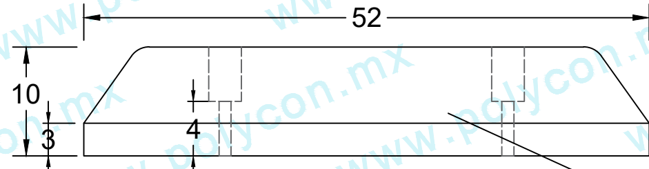
VISTA LATERAL
