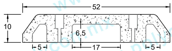
CORTE A-A'
