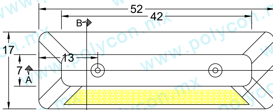
VISTA SUPERIOR
