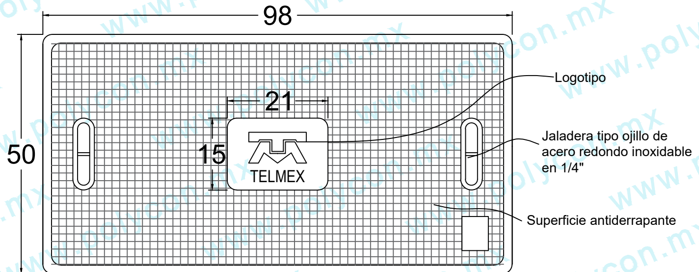
VISTA SUPERIOR
