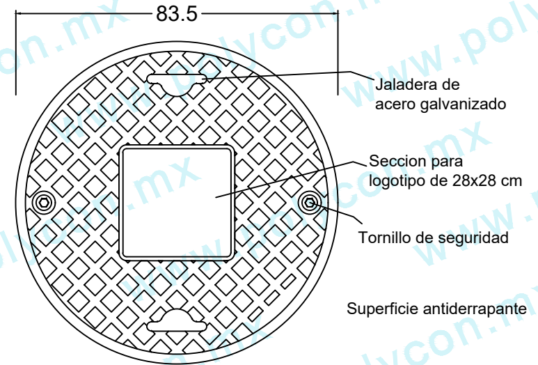
VISTA SUPERIOR
