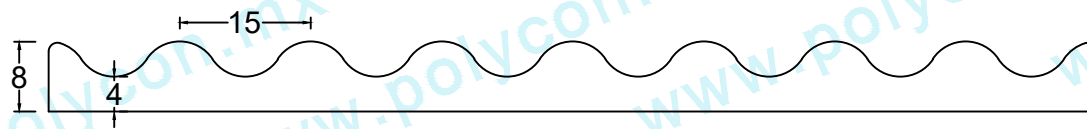
VISTA LATERAL
