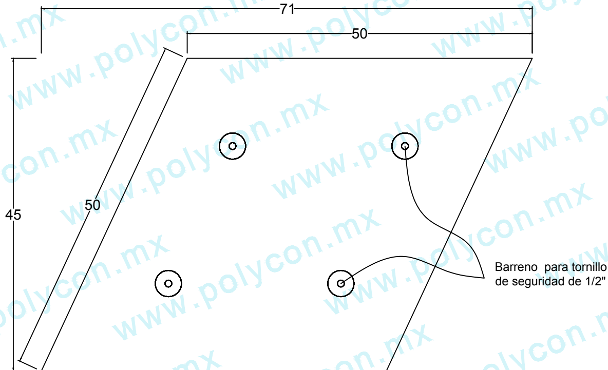
VISTA SUPERIOR
